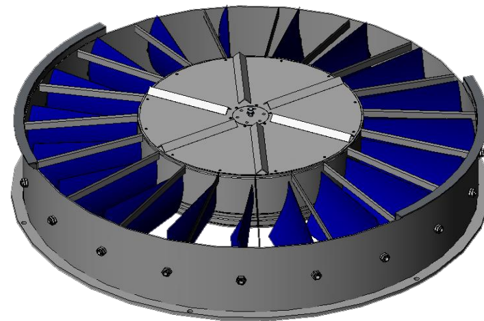
Спрямляющий аппарат
